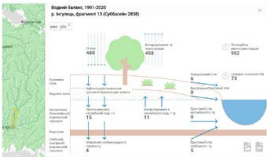
Рис. 2.4. Схема водного балансу ділянки р. Інгулець
