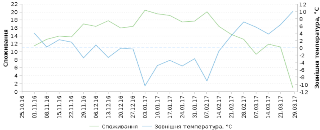
Динаміка споживання та градусо-днів Тепло, Гкал
